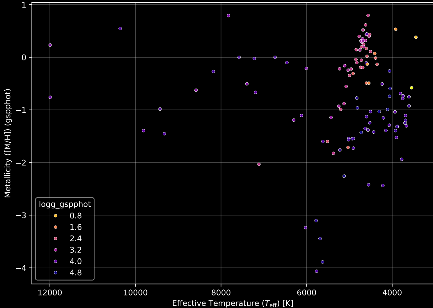
APOGEE DR17 Field: [005+02-O] Stellar Population Parameters (n= 117)
